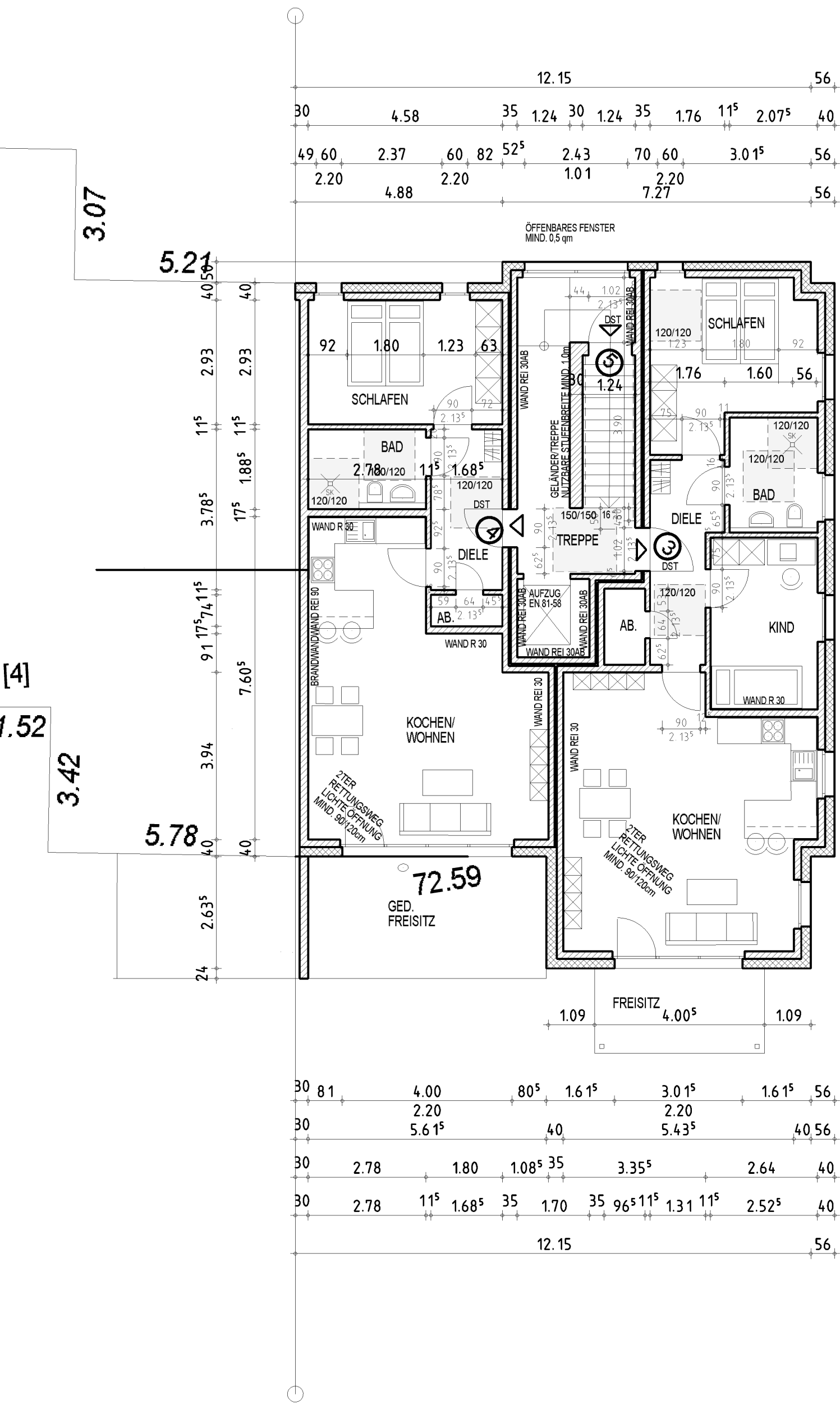
OBERGESCHOSS HAUS B
